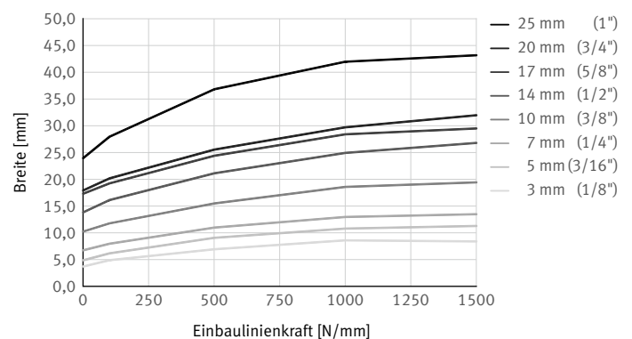
GORE® Schnurdichtung - Verpressungskennlinien bei Raumtemperatur
